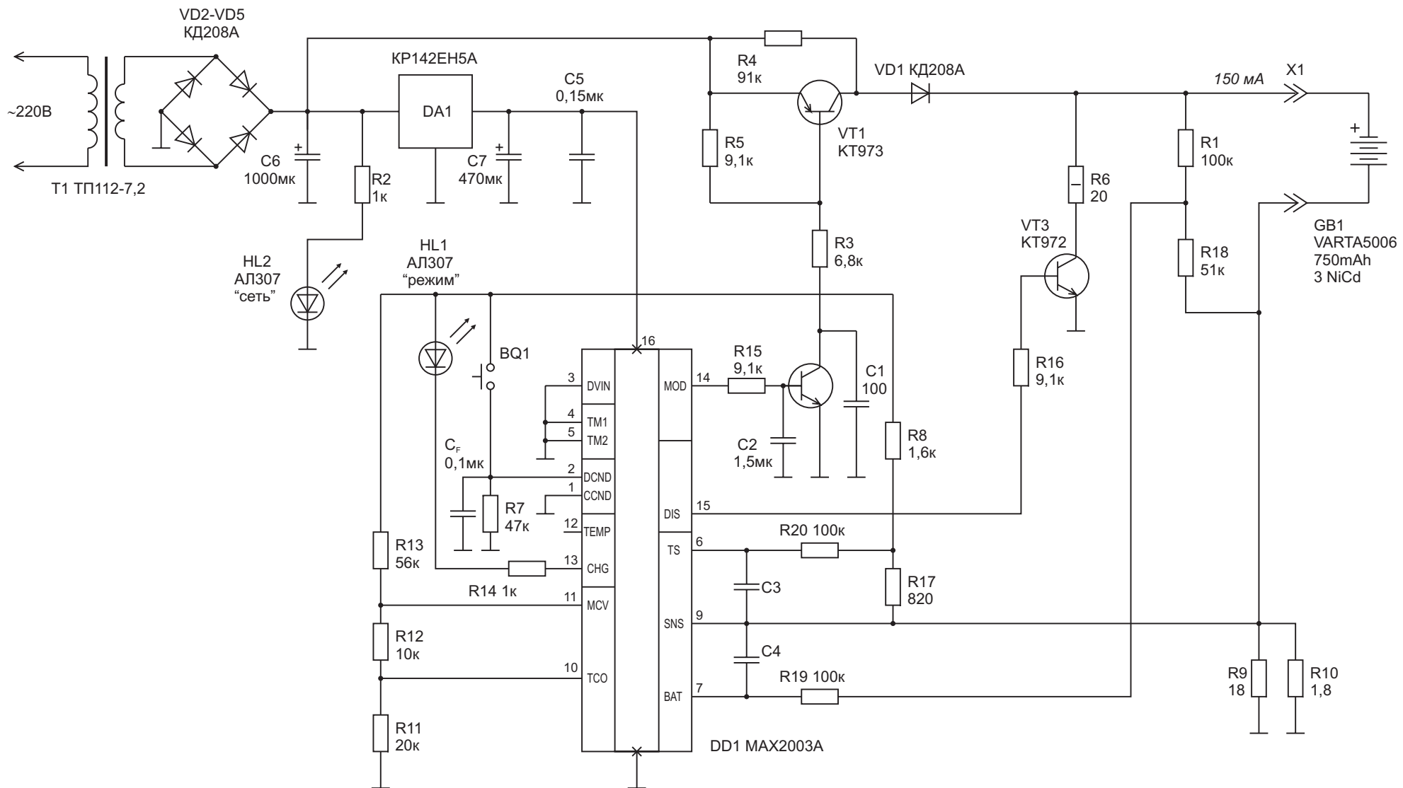
УЗ36.00.00.000 ЭЗ. Схема электрическая принципиальная устройства зарядного УЗ-3,6-А.
