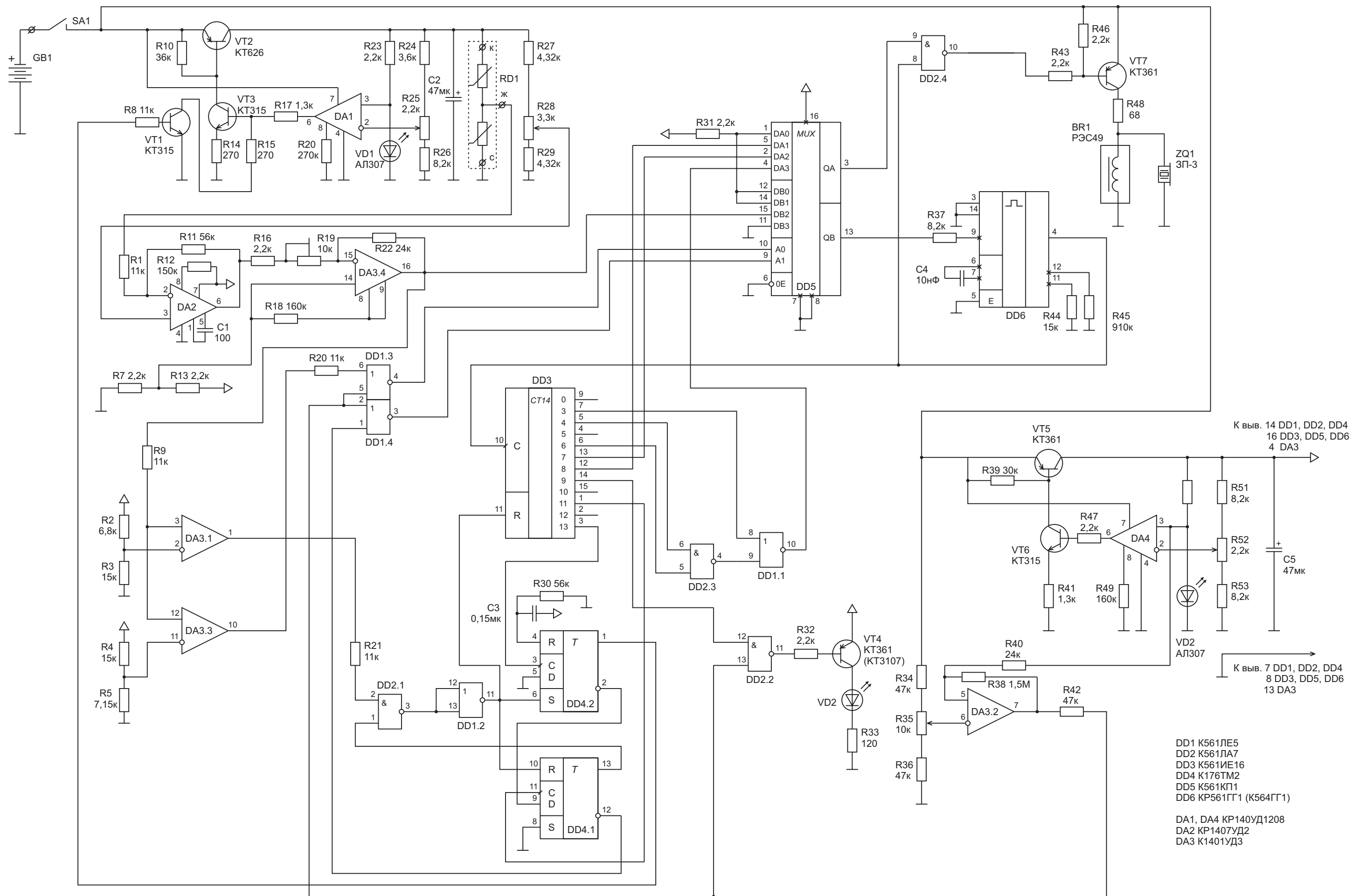
TM.00.00.000 Э3. Течеискатель ЛЮКС TM-1. Схема электрическая принципиальная.
