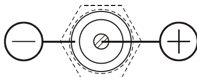
Рисунок 4 – Полярность гнезда для подключения адаптера
