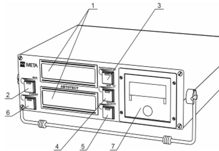
1-Индикаторы; 2-Кнопка включения питания ВКЛ; 3-Кнопка РАБОТА/ПАУЗА; 4-Кнопка КОР.0; 5-Кнопка ПЕЧАТЬ; 6-Кнопка РЕЖИМ; 7- Принтер
