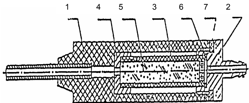
1-Рукоятка; 2-Штуцер; 3-Патрон; 4-Крышка патрона; 5-Фильтрующий агент (стекловолокно); 6,7-Прокладка
